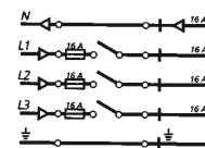
Schaltbild mit 3 Zuleitungen:
