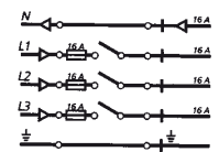
Schaltbild mit 3 Zuleitungen:
